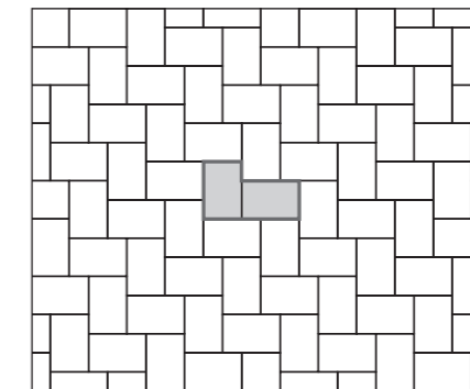
VERLEGEMUSTER F
