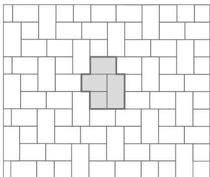
VERLEGEMUSTER S
