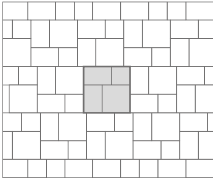
VERLEGEMUSTER P
