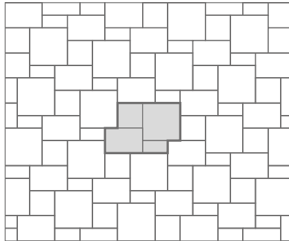
VERLEGEMUSTER Q
